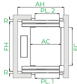
2 wejścia (przelotowe)
