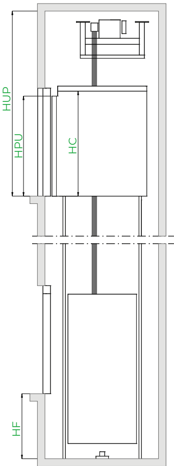
Verticale doorsnede
