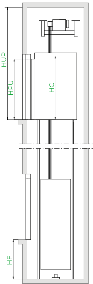
Sección vertical
