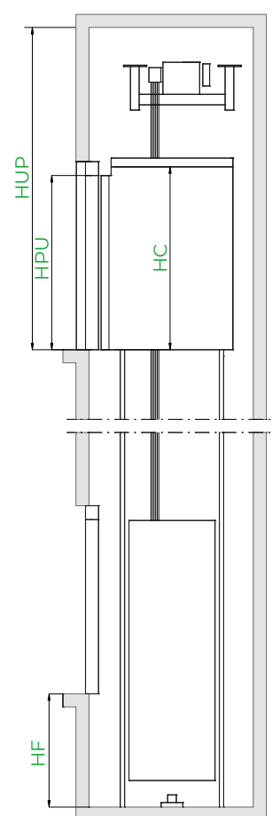
Sección vertical
