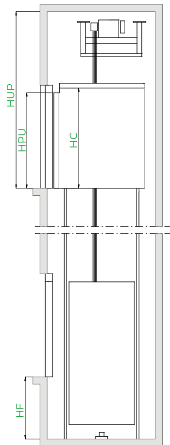
Sección vertical
